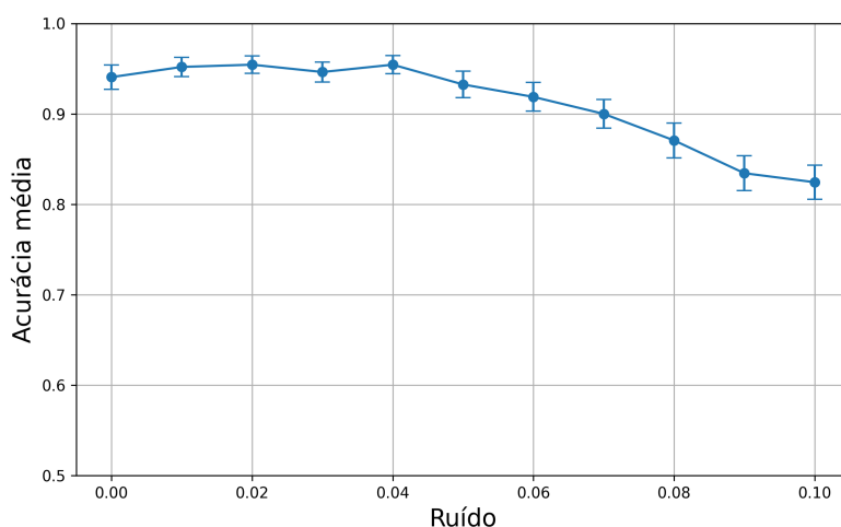
Figura 4. Acurácia do modelo global em função do nível de ruído.
