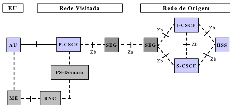
Figura 1: Arquitetura de Segurança entre Domínios Seguros
