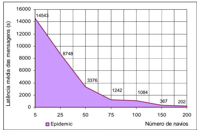
Figura 9. Latência da rede.
