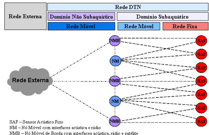
Figura 4. Comunicação entre nós móveis e sensores.
