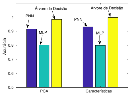
(a) Acurácia da classificação.
