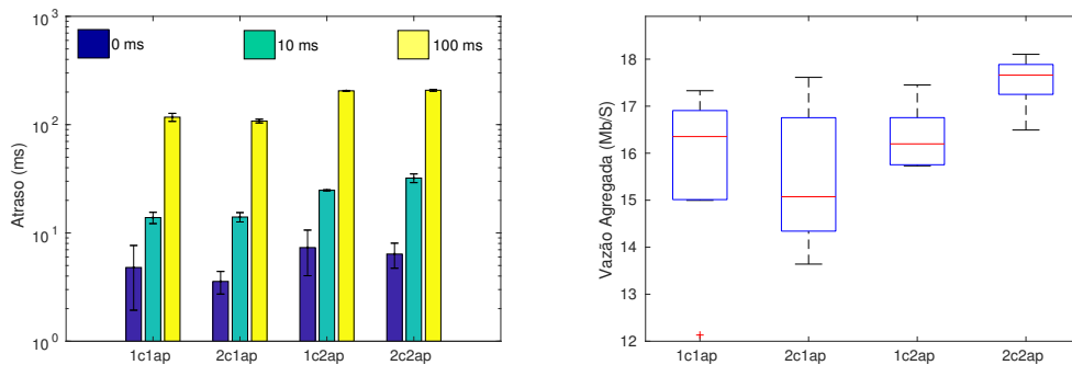
(a) Atraso com virtualização do sem-fio.
