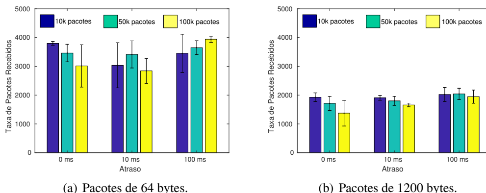
Figura 3. Taxa de pacotes de recebidas pelo consumidor de dados ao realizar envios em taxas superiores à capacidade do enlace sem-fio. O atraso entre o gateway e a infraestrutura de virtualização de rede não influencia nas taxas alcançadas. Os experimentos foram realizados com fluxos UDP com pacotes pequenos (a) 64 bytes e pacotes grandes (b) 1200 bytes.
