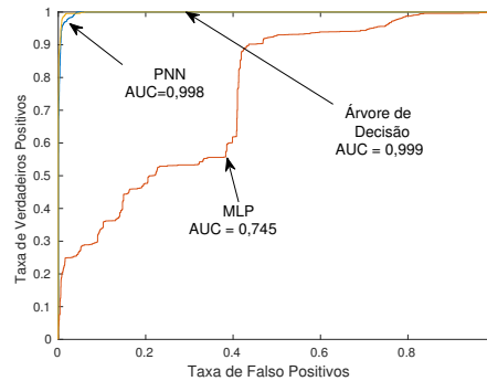
(b) Curva ROC para a classe de ataque.
