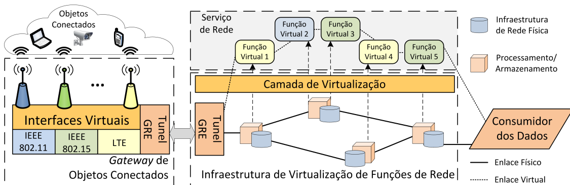
Figura 2. A infraestrutura de virtualização de funções de rede para Internet das Coisas. O Gateway de Objetos Conectados abstrai o método de acesso através de interfaces virtuais conectadas por túnel à Infraestrutura de Virtualização de Funções de Rede (NFVI). O gateway envia os quadros diretamente para a NFVI.
