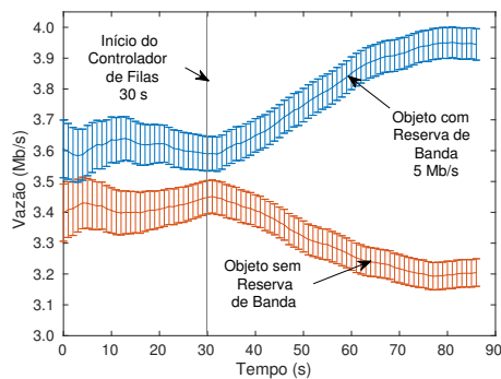
(a) Diferenciação entre fluxos.
