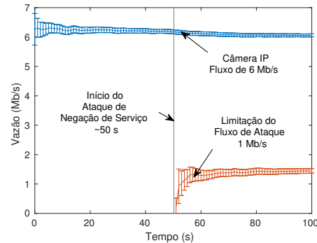
(b) Ataque de negação de serviço na rede.
