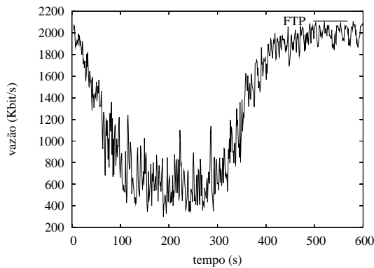
Figura 5.6: Vazão Agregada do Tráfego FTP sem Controle de Carga
