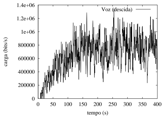
Figura 5.2: Carga do tráfego agregado de voz no sentido de descida, medida pelo estimador no AP em cada intervalo de amostra.
