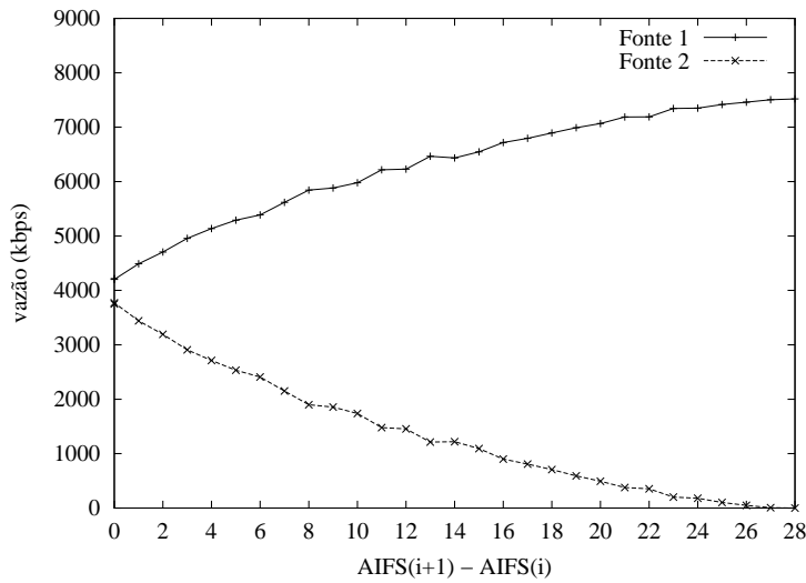
Figura 4.10: Vazão de Duas Fontes de Categorias Distintas em Função da Sobreposição de Janelas
