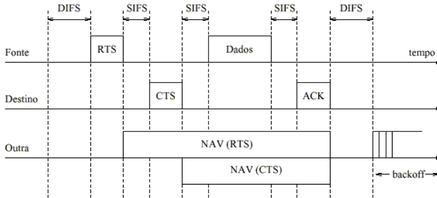
Figura 2.4: Acesso DCF com RTS / CTS.
