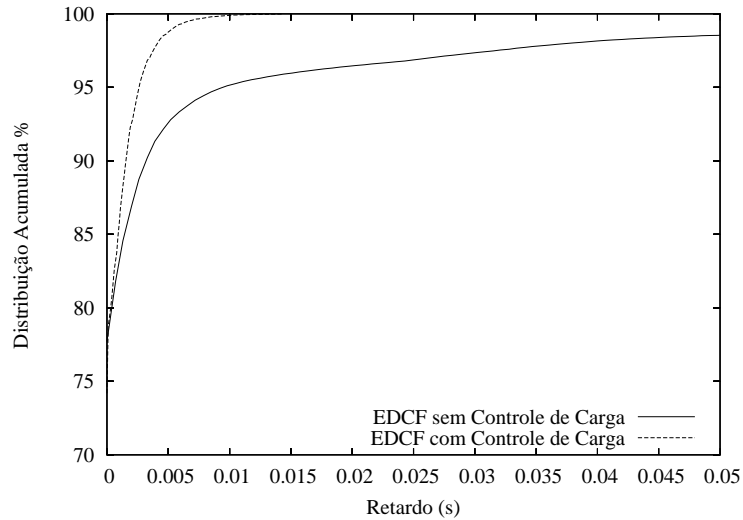
Figura 5.5: Distribuição do Retardo do Tráfego de Tempo Real
