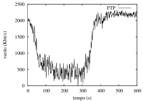
Figura 5.7: Vazão Agregada do Tráfego FTP com Controle de Carga
