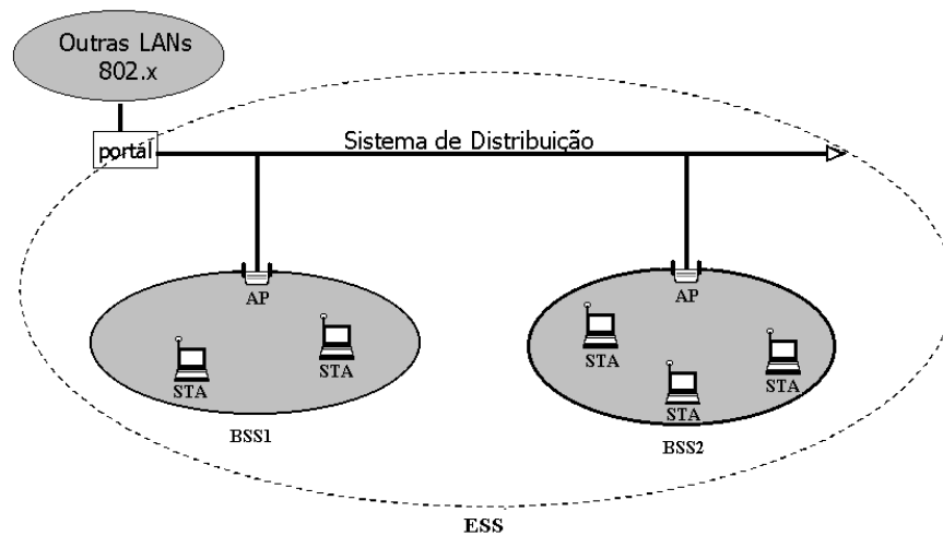
Figura 2.1: Componentes de uma Rede 802.11 Infra-Estruturada
