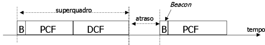
Figura 2.5: Superquadro e Divisão de Períodos (CP e CFP).
