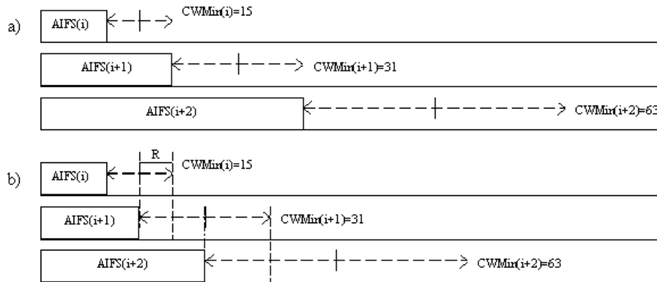
Figura 4.9: Diferenciação por Variação Conjunta de AIFS e CWMin
