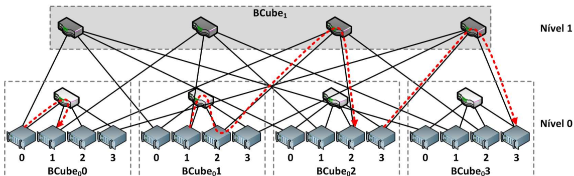
Figura 2. Topologia utilizada pela arquitetura BCube.
